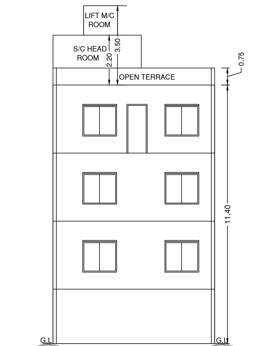
ELEVATION
